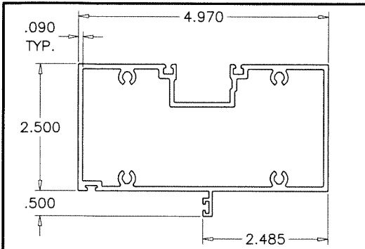
E1 DOOR HEADER Series 9000
