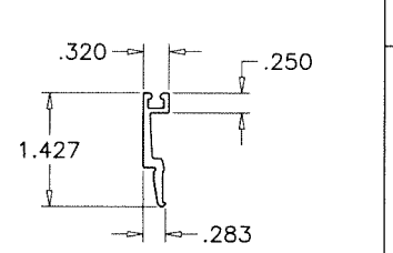
E20 DOOR SWEEP
