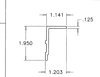
E14 LOCK BACK UP PLATE
