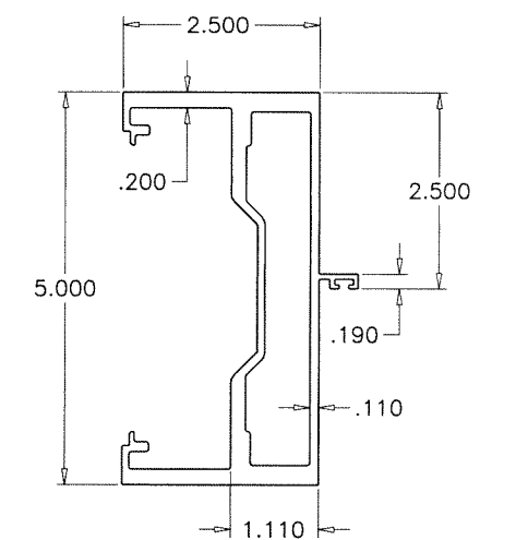
E3 DOOR JAMB Series 9000
