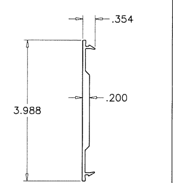
E15 JAMB FILLER
