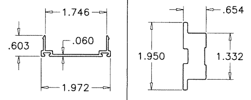
E20 DOOR SWEEP
